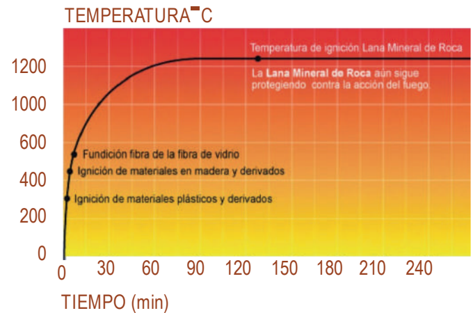
COMPORTAMIENTO DE MATERIALES EN EL FUEGO CURVA NORMALIZADA ISO 834
