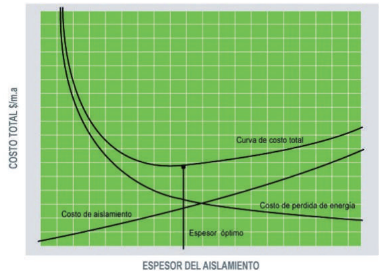
Curva termoeconómica Espesor vs Costo
