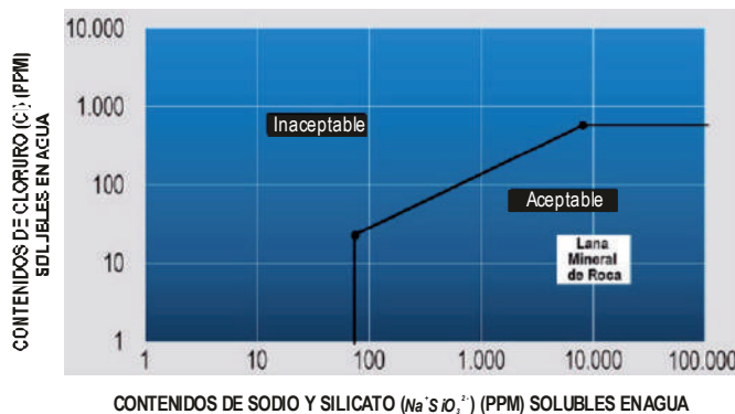
ANÁLISIS DE ACEPTABILIDAD DE UN MATERIAL AISLANTE EN FUNCIÓN DE SU COMPOSICIÓN EN IONES Cl, Na + y SiO 2 +
